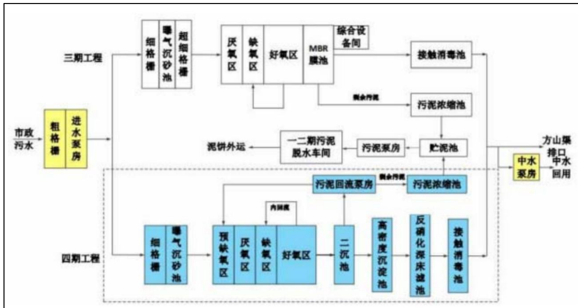
图 4-2 江宁科学园污水处理厂三期工艺流程图
