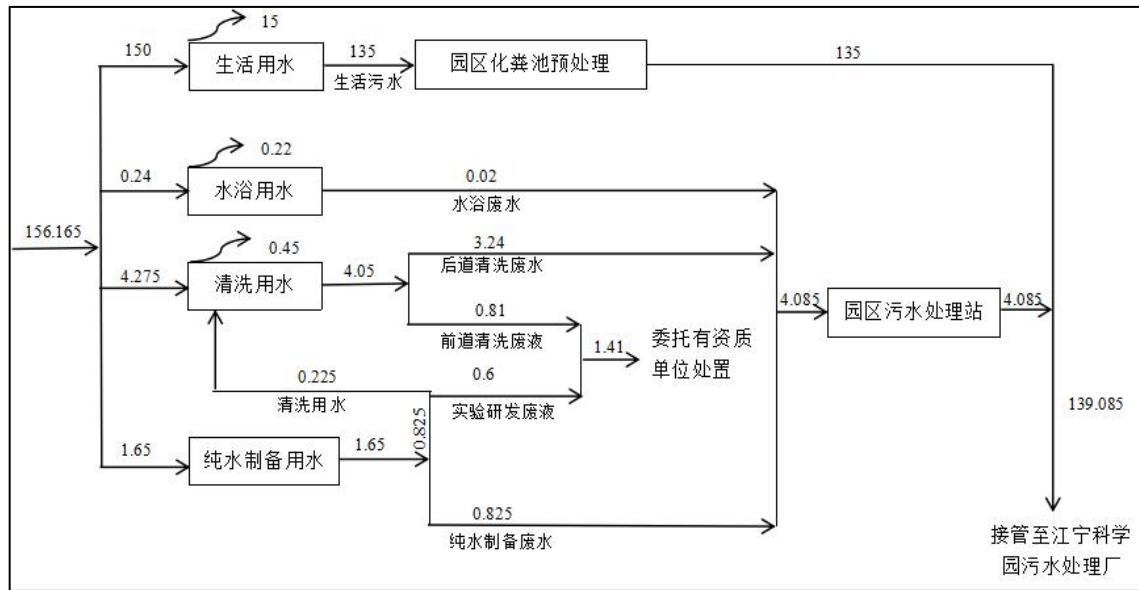
图 2-1 全厂水平衡图（单位：m 3 /a）
