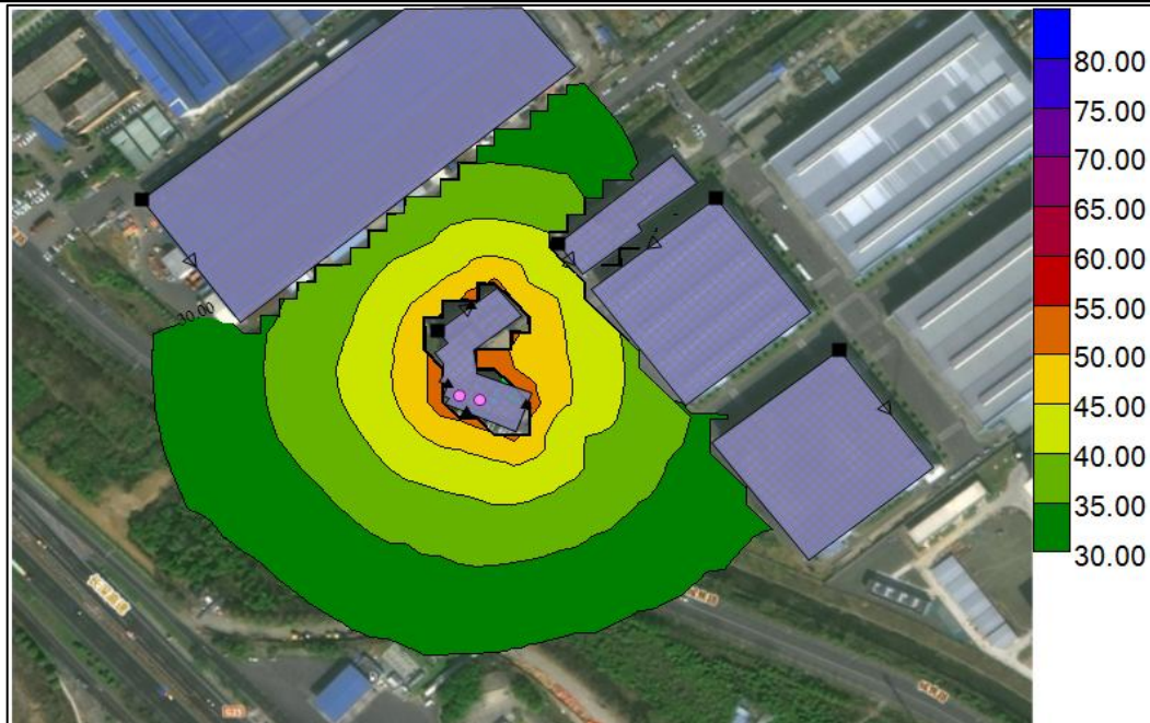
图 4-3 企业厂界噪声预测结果等值线图
